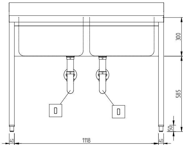
Oldalnézet
